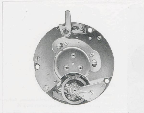
Platinen 45 mm
