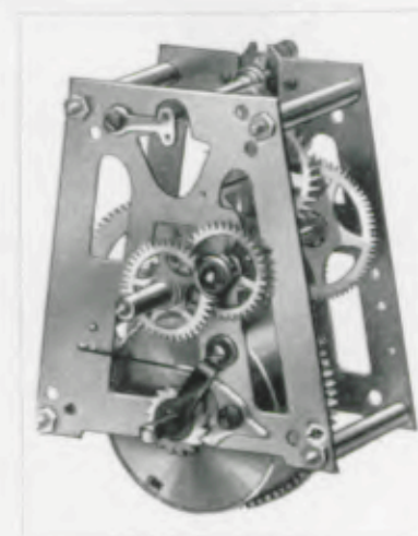
Werk Nr. 74 Platinen 8,5 x 8,2 cm 14 Tag Pendelgehwerk
