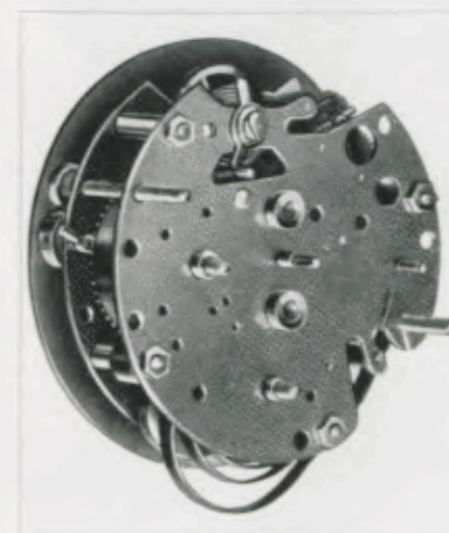
Werk Nr. 81 Platinen 54 x 54 mm Zuverlässiges, flaches Weckerwerk, Schlag auf Werkkapsel.
