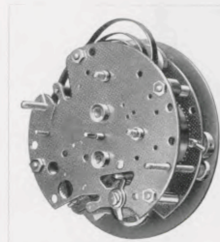
Werk Nr. 81 Platinen 54 x 54 mm Zuverlässiges, flaches Weckerwerk, Schlag auf Werkkapsel
