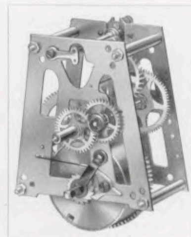
Platinen 8,5 x 8,2 cm 14 Tag Pendelgehwerk
