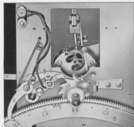
Signalvorrichtung bei der ATO-Signaluhr 8010
