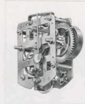
Werk Nr. 231 7,1 x 5,6 cm Normalwerk, große Balance
