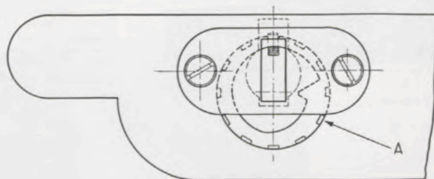
Aufhängevorrichtung der Konsole. D. R. P. A.
