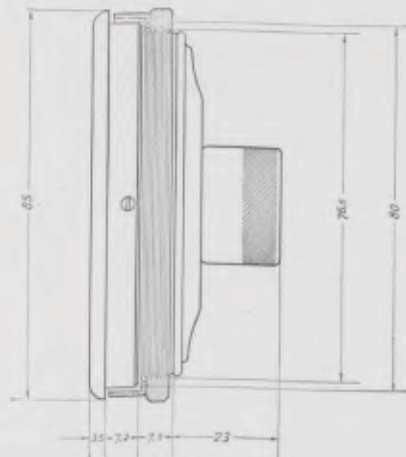
80 mm Einpaß — 80 mm opening — 80 mm emboltage — 80 mm diámetro de acoplamiento
