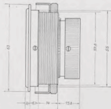
55 mm Einpaß — 55 mm opening — 55 mm emboltage — 55 mm diámetro de acoplamiento
