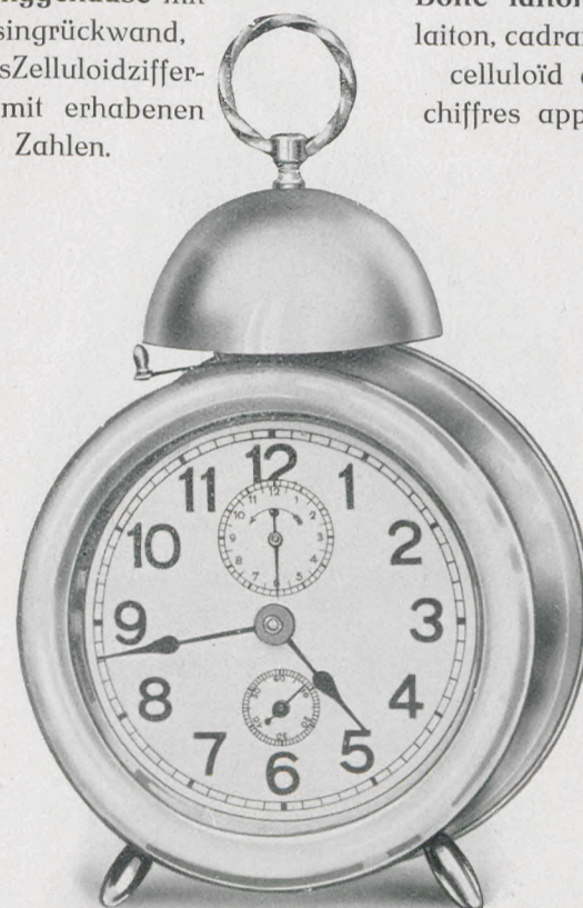
21 cm No. 7952 Vernickelt — Nickelé } 1 Tag Wecker. „ 7976 Verkupfert — Cuivré } „ 7977 Königsrot — Pourpre de roi } 30 heures réveil.
