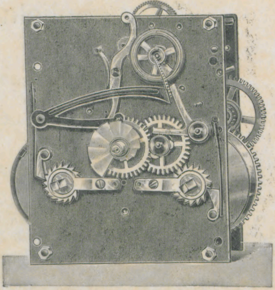
Auslöser für Stundenschlag.
