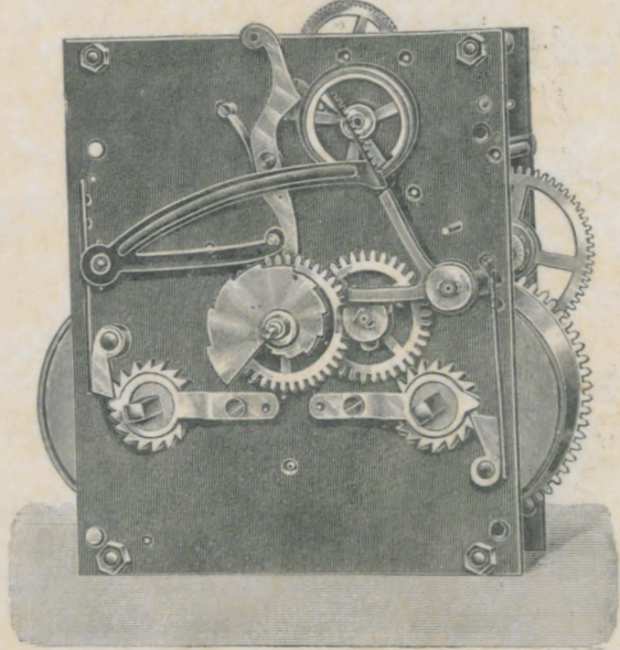
Auslöser für Halbschlag.
