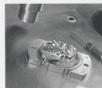
Verzieren der Werkbrücken mit Dekorschleifen. Decorating the movement bridges with grinding finish.
